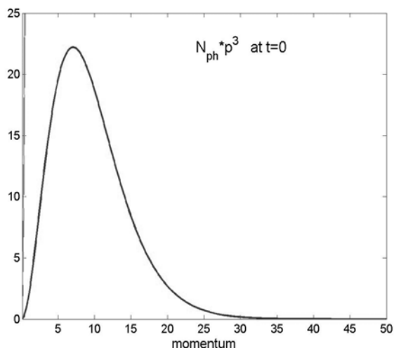
Рис. 4. Зависимость произведения термодинамически равновесной функции распределения фононов (функция Бозе-Эйнштейна (в момент времени t=0 )) на куб импульса от безразмерного импульса
